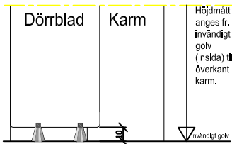
Alternativ 7 Utåtgående
