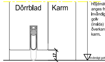
Alternativ 8 Utåtgående
