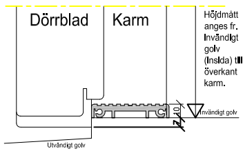
Alternativ 4 Utåtgående
