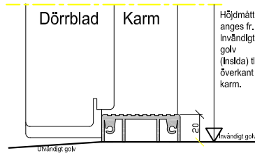
Alternativ 5 Utåtgående
