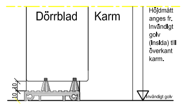
Alternativ 6 Utåtgående
